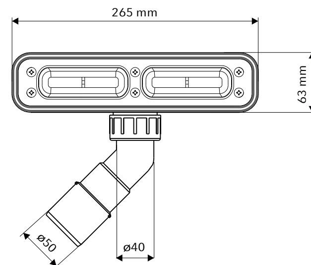
Pohľad zhora
