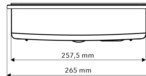
Pohľad predný
